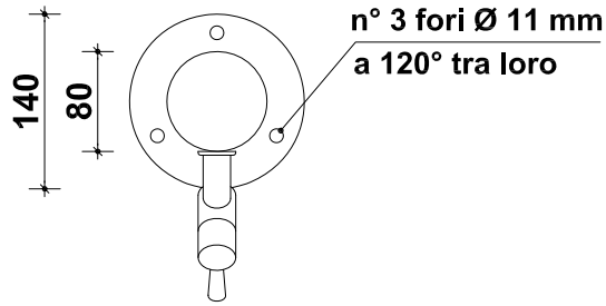
prospetto frontale
