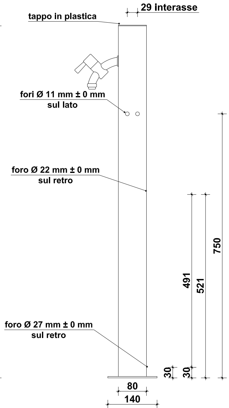
prospetto laterale
